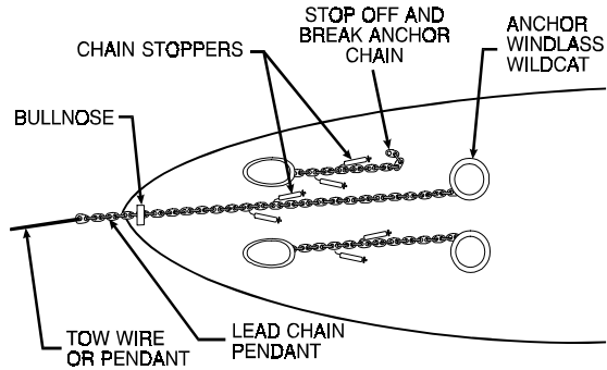
Figure 6-5. Pendant or Single-Leg Rig.
